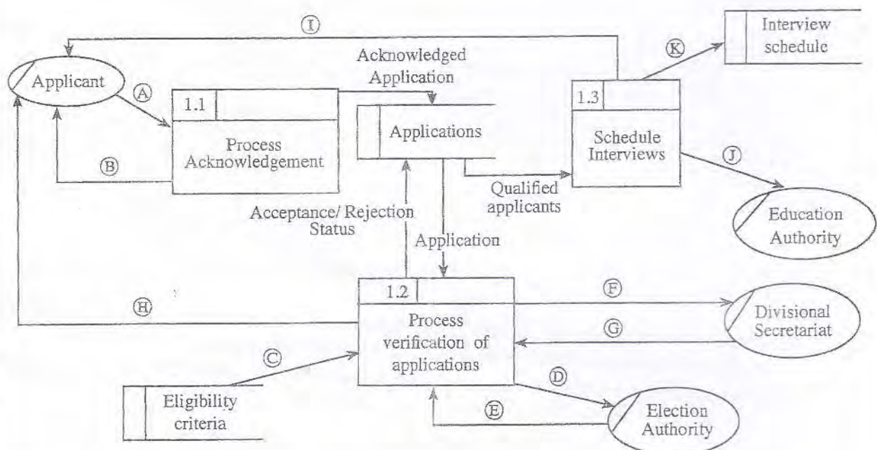
Level 1 DFD
